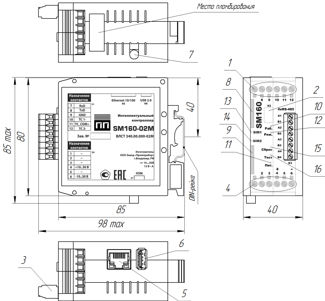
Рисунок А.1 – Общий вид контроллера
