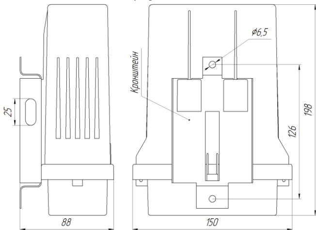
Рисунок Б.1 – Внешний вид и размеры счетчика в исполнении С
