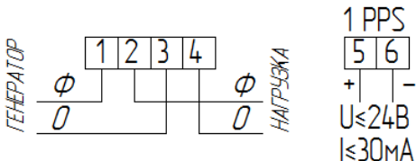
Рисунок А.1 - Схема подключения счетчика в исполнении С
