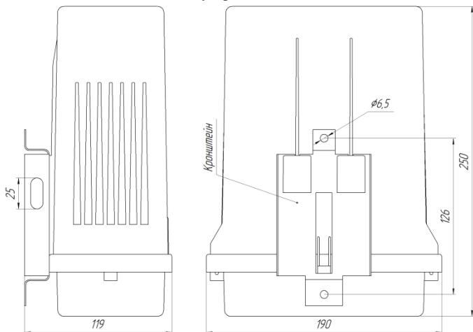
Рисунок Б.1 – Внешний вид и размеры счетчика в исполнении С
