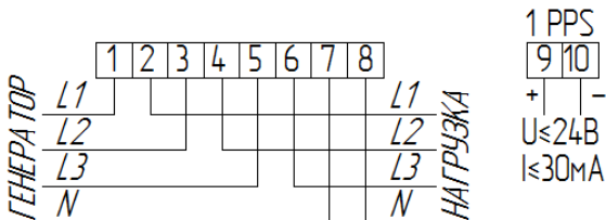
Рисунок А.1 - Схема подключения счетчика в исполнении С
