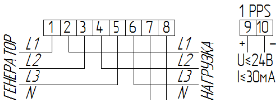
Рисунок Б.1 - Схема подключения счетчика в исполнении С
