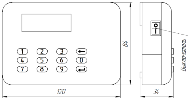
Рисунок Б.2 - Внешний вид и размеры индикаторного устройства
