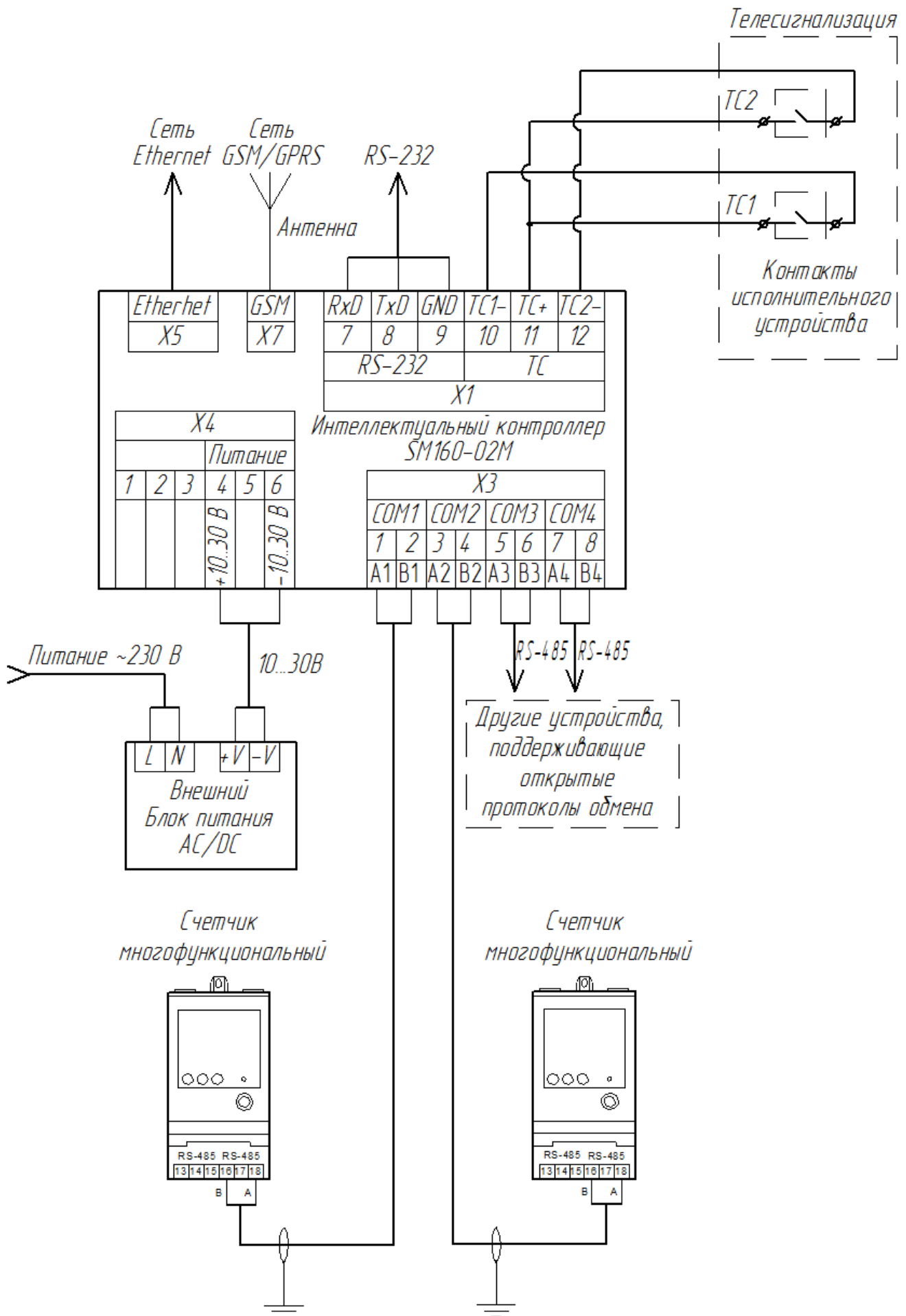
Рисунок Б.1 – Пример подключения внешних цепей контроллера
