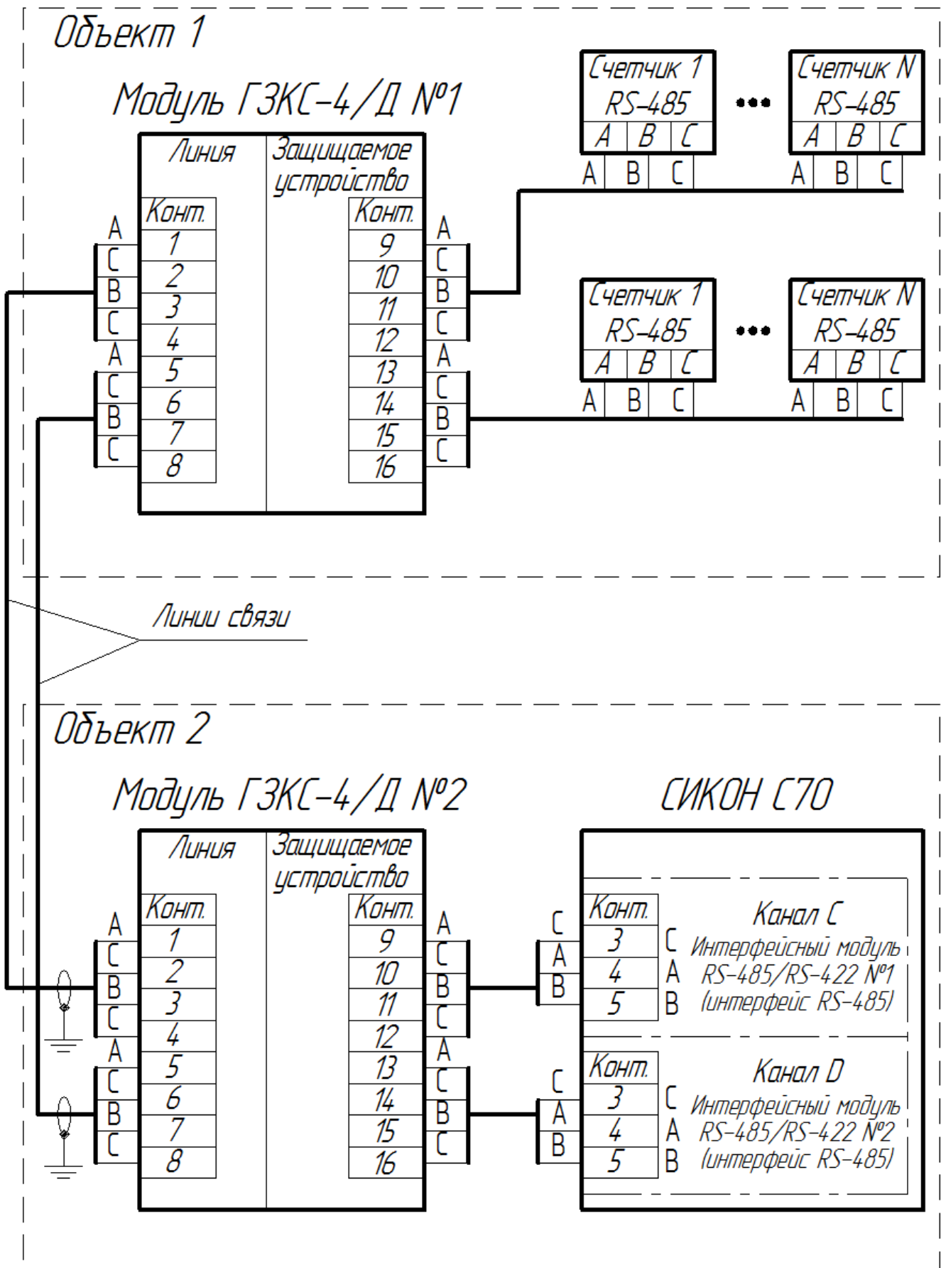
Рисунок Б.3 – Пример использования модулей грозозащиты ГЗКС-4/Д (защита двух линий) для подключения счетчиков к контроллеру СИКОН С70 по интерфейсу RS-485 (А, В, С)
