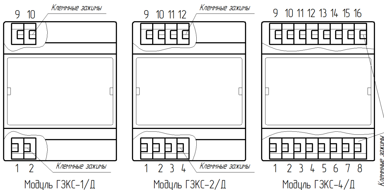
Рисунок А.2 – Модули грозозащиты различных модификаций со снятыми крышками
