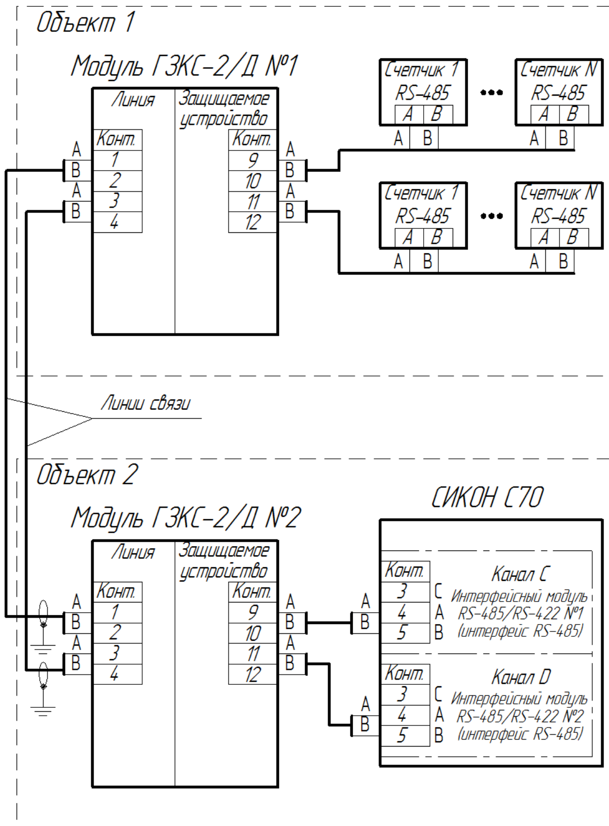
Рисунок Б.2 – Пример использования модулей грозозащиты ГЗКС-2/Д (защита двух линий) для подключения счетчиков к контроллеру СИКОН С70 по интерфейсу RS-485 (А, В)
