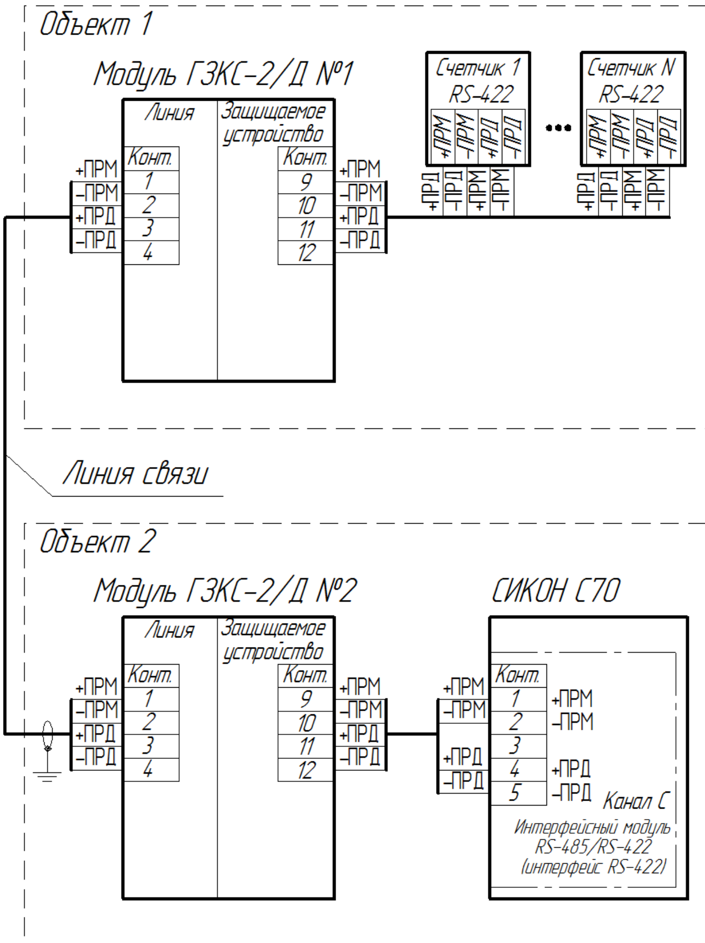
Рисунок Б.1 – Пример использования модулей грозозащиты ГЗКС-2/Д для подключения счетчиков к контроллеру СИКОН С70 по интерфейсу RS-422
