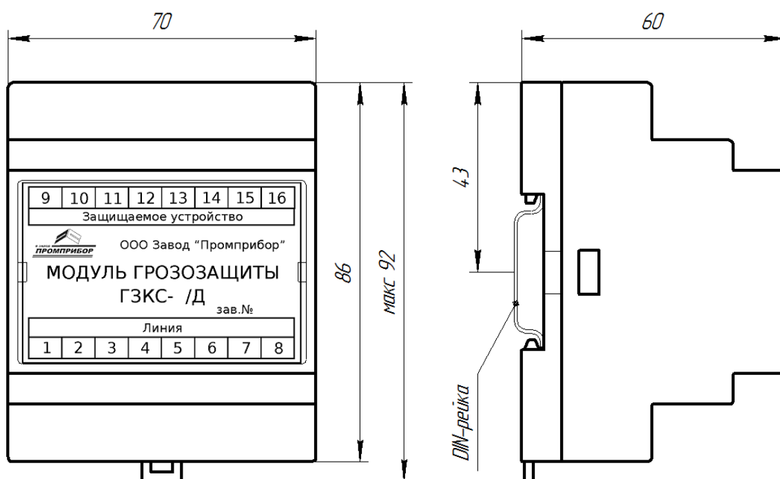
Рисунок А.1 – Габаритные и установочные размеры модуля грозозащиты
