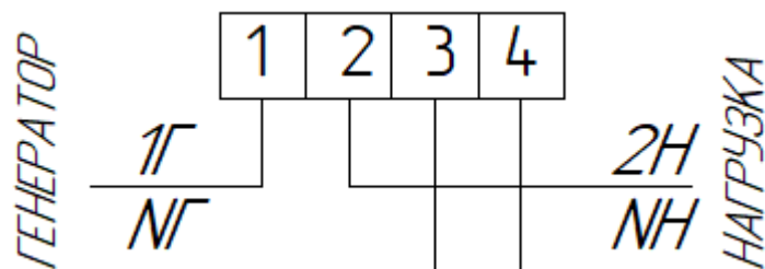
Рисунок А.3 - Схема подключения счетчика в исполнении С
