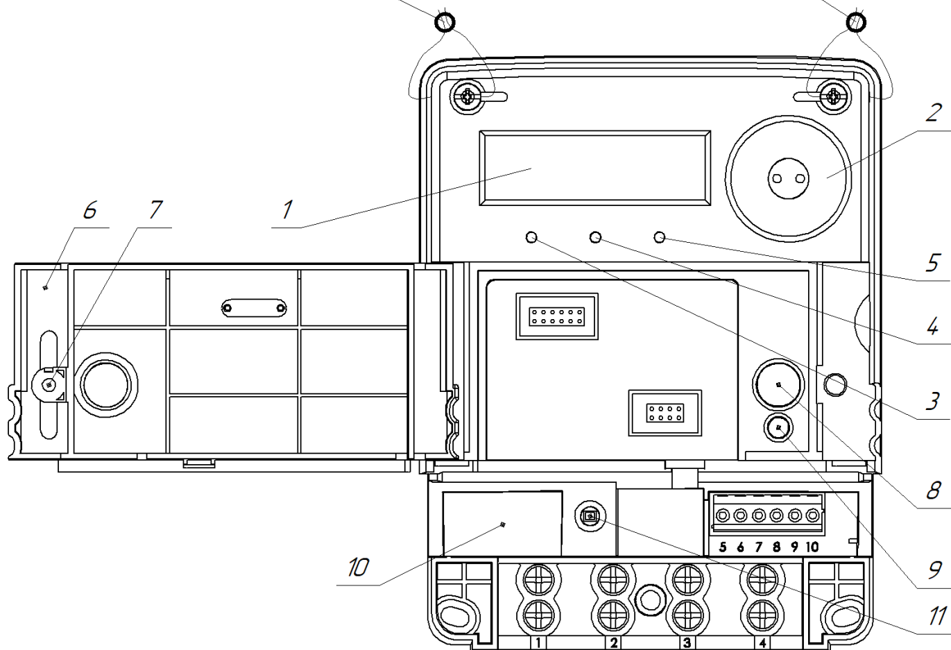
Рисунок А.2 - Счетчик в исполнении W со снятой крышкой клеммной колодки и открытой крышкой отсека сменного связи
