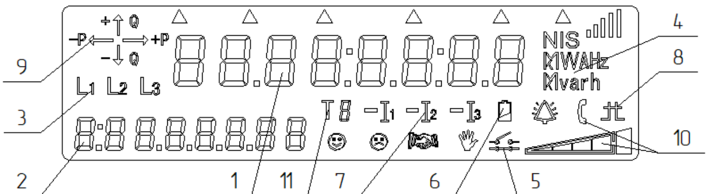
Рисунок Б.1 – Общий вид дисплея счетчика
