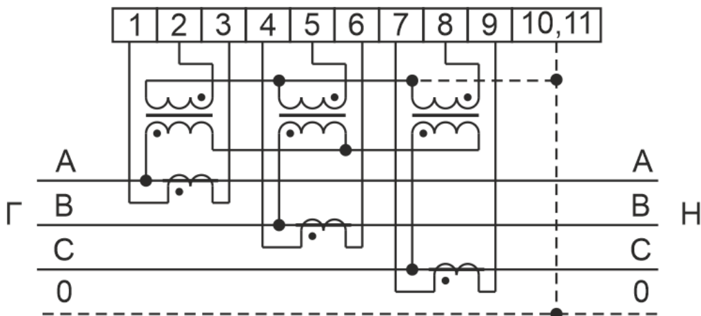
Рисунок А.2 - Схема подключения счетчика косвенного включения в исполнении W с помощью трех трансформаторов тока и трех трансформаторов напряжения
