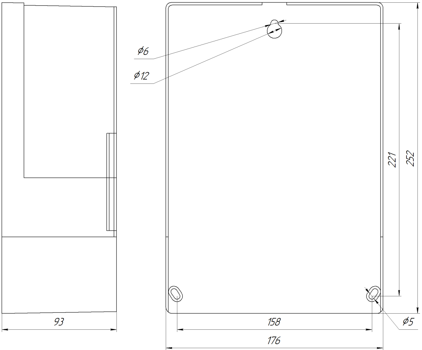
Рисунок А.1 - Размеры счетчика косвенного включения в исполнении W
