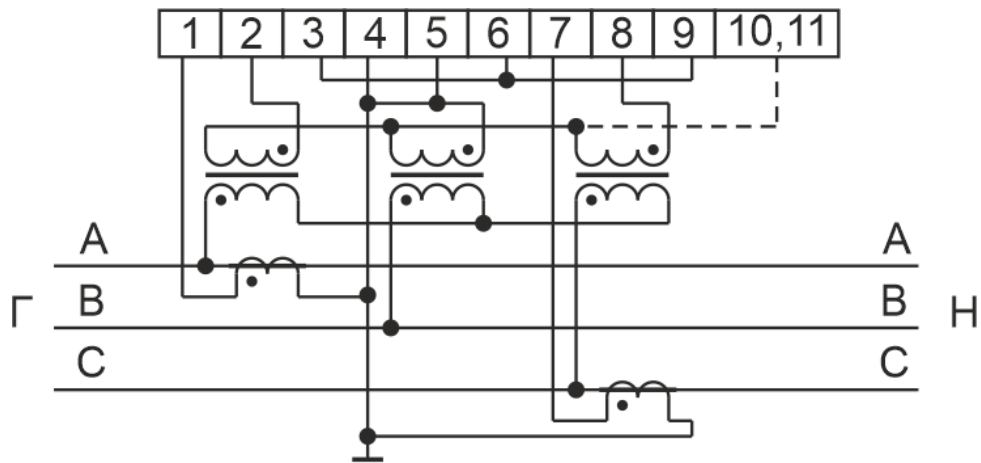
Рисунок А.3 - Схема подключения счетчика косвенного включения в исполнении W с помощью двух трансформаторов тока и трех трансформаторов напряжения
