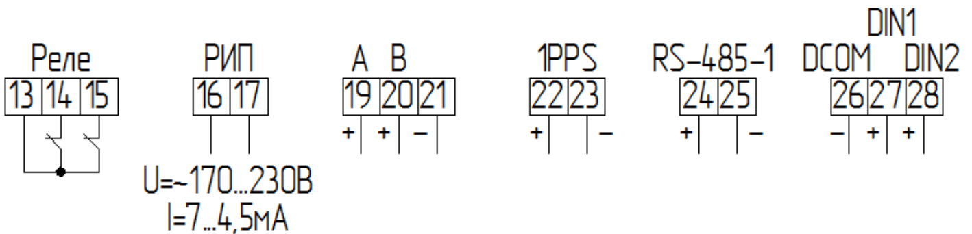
Рисунок А.4 – Подключение сигнальных цепей счетчика косвенного включения в исполнении W (назначение групп контактов слева направо: два дискретных выхода; резервный источник питания; активная/реактивная энергия; выход 1PPS; интерфейс RS-485 линия A «+» и линия B «-»; два дискретных входа)
