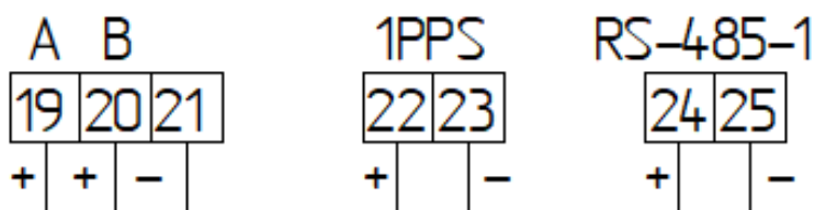
Рисунок А.3 – Подключение сигнальных цепей счетчика непосредственного включения в исполнении W (назначение групп контактов слева направо: активная/реактивная энергия; выход 1PPS; интерфейс RS-485 линия A «+» и линия B «-»)
