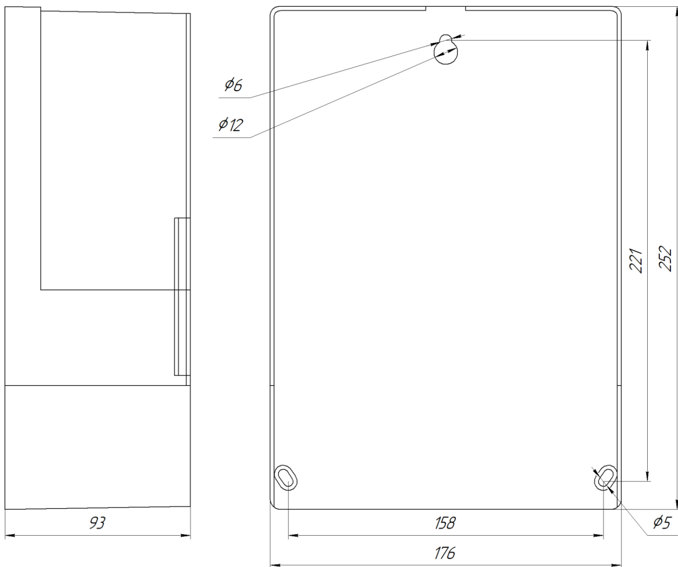
Рисунок А.1 - Размеры счетчика непосредственного включения в исполнении W
